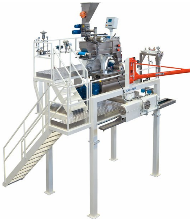
■ Presse automatique 130.1-1500/1 TV/L
