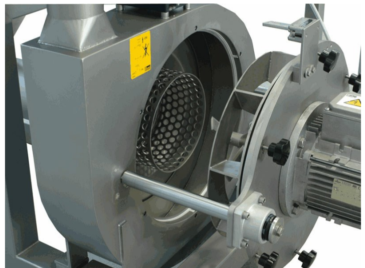
Detalle triturador abierto
