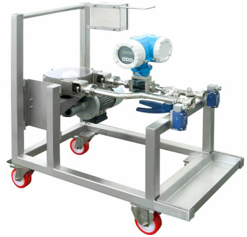
■ Pompa peristaltica carrellata
