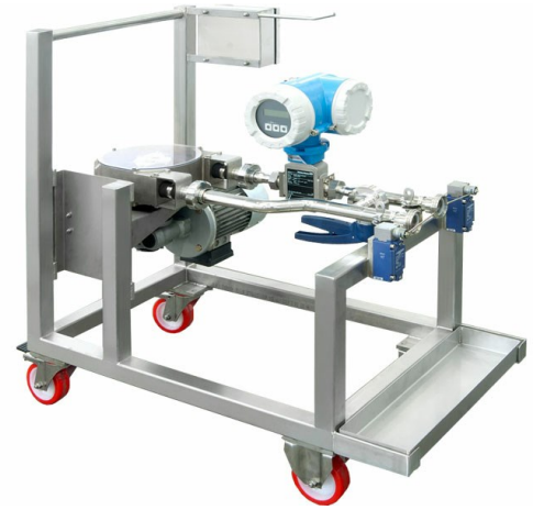
■ Pompe péristaltique sur chariot
