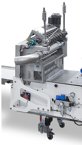
Formeuse de lasagne
