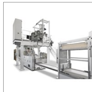
Dettaglio pressa 180.1
